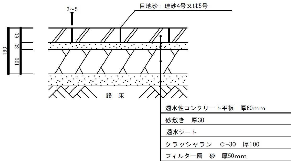
図 5.3 一般歩道部透水性舗装(区分 1)
