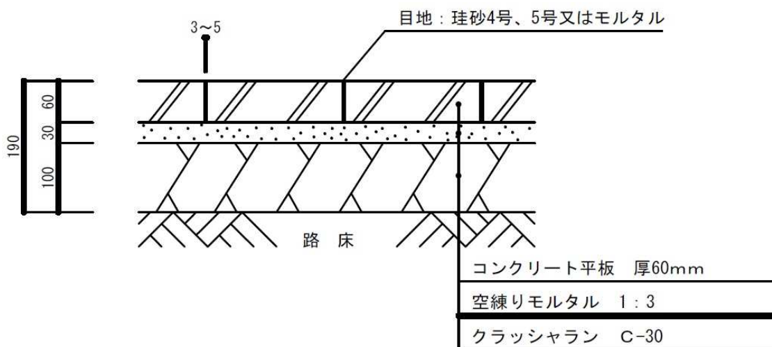
図 5.1 一般歩道部普通舗装(区分 1)
