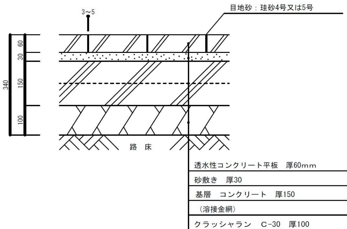
図 5.5 車両乗入れ部排水性舗装(1種)
