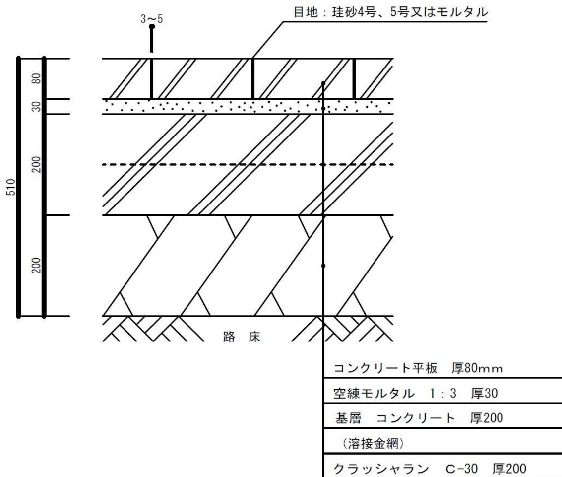
図 5.4 車両乗入れ部普通舗装(2種)
