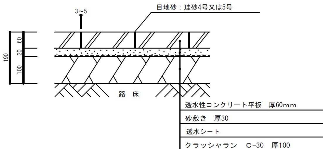
図 5.2 一般歩道部排水性舗装(区分 1)
